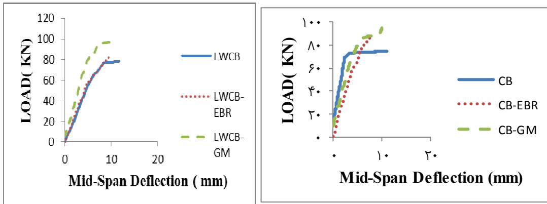
ب) تیرهای بتن معمولی و بتن سبک فاقد الیاف در مطالعه مدن دوست و رحیمی [۲۷] شکل ۳-۴: نمودار بار - خیز وسط دهانه تیرهای بتن مسلح معمولی و سبک
