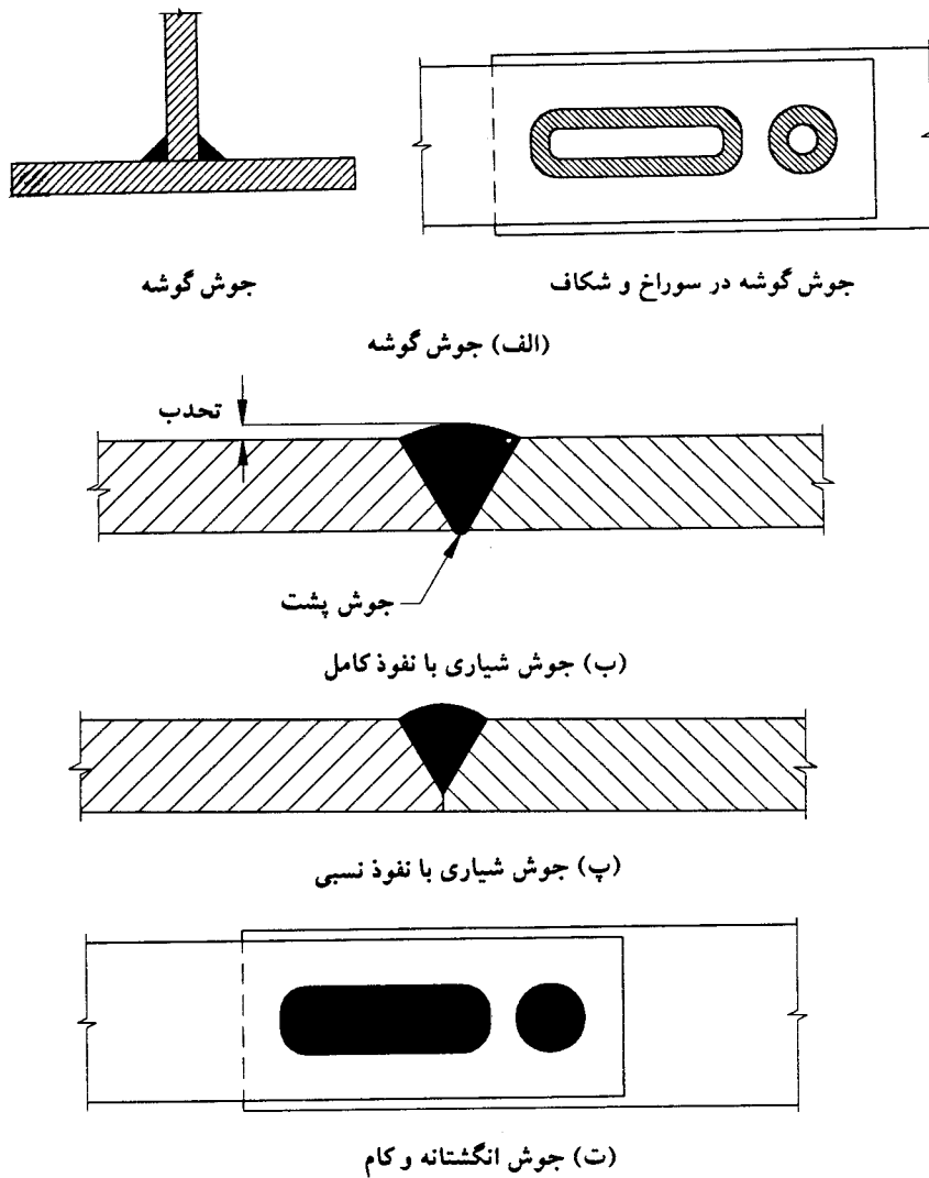
شکل ۱-۱ انواع جوش.
